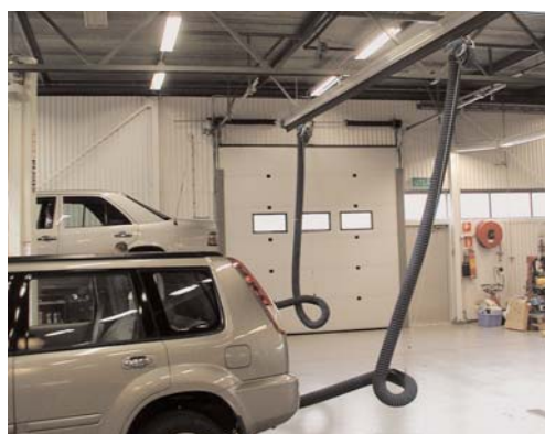
Gruppo aspirante Blindotubo 920/400.
